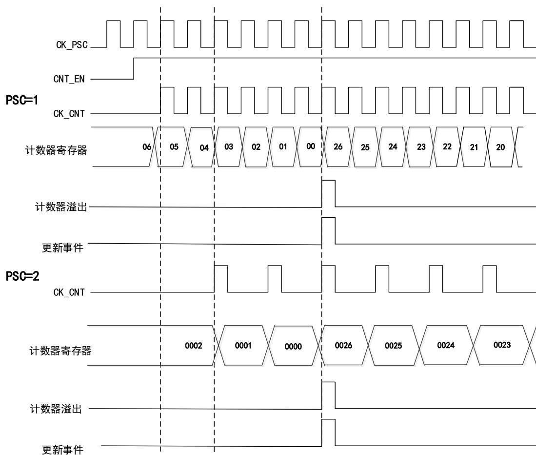
图 69 向下计数模式下，分频因子为 1 或 2 的时序图
