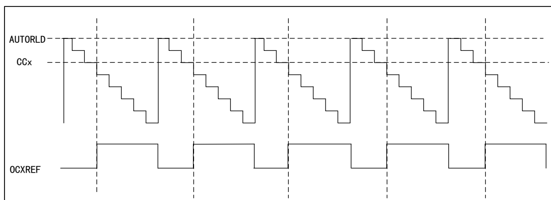
图 46 PWM1 向下计数模式的时序图
