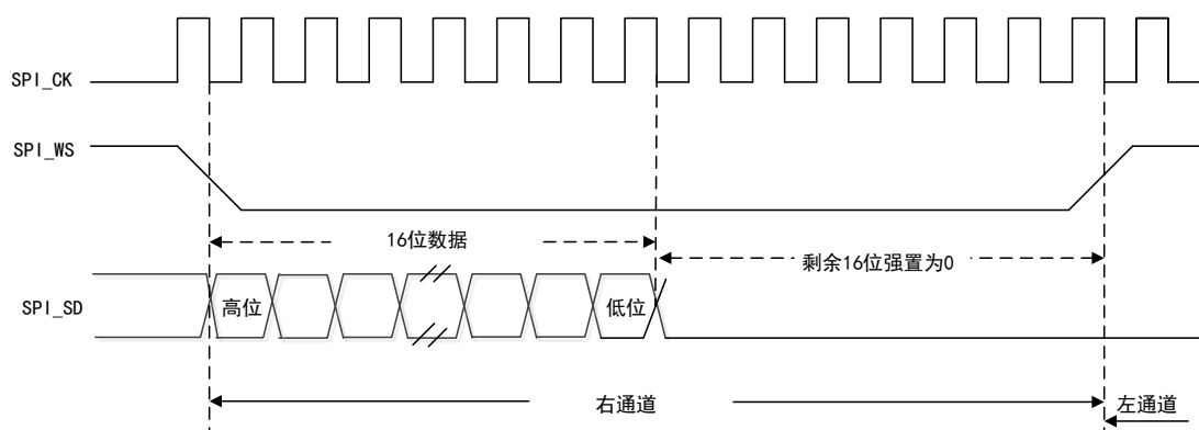
图 118 MSB 对齐标准波形（16 位扩展至 32 位）
