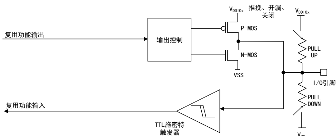
图 22 复用模式下的 I/O 结构
