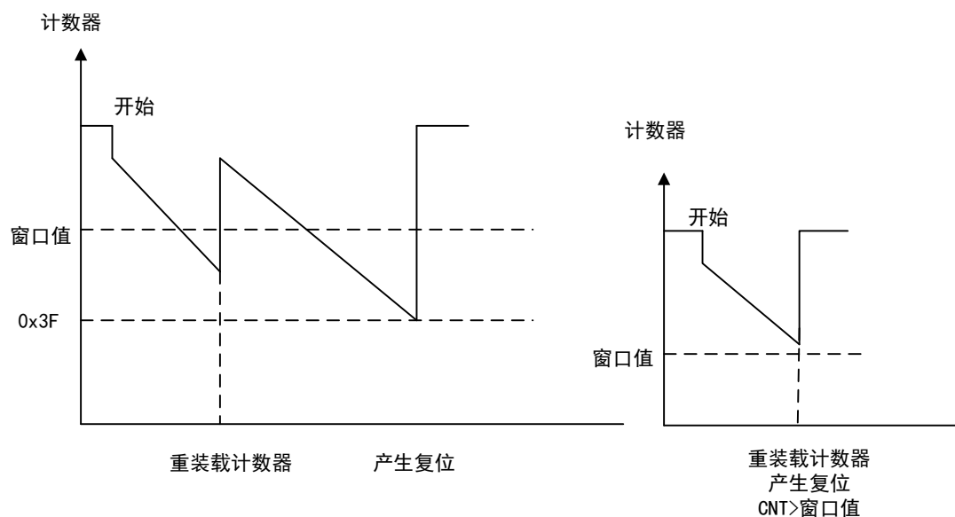
图 90 窗口看门狗时序图
