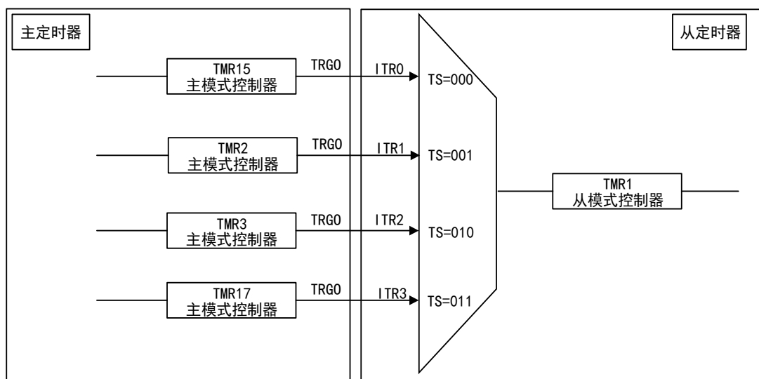
图 85 定时器 1 主/从模式的例子
