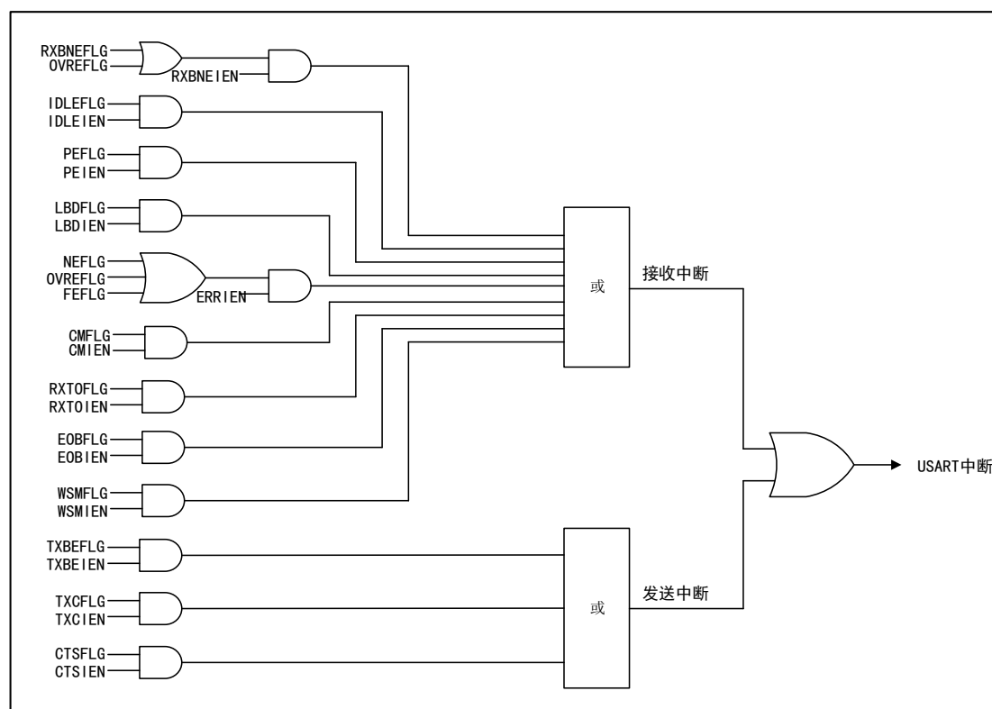
图 102 USART 中断映射
