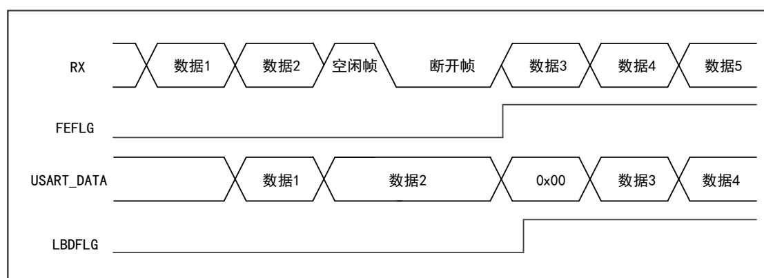
图 97 空闲状态检测断开帧
