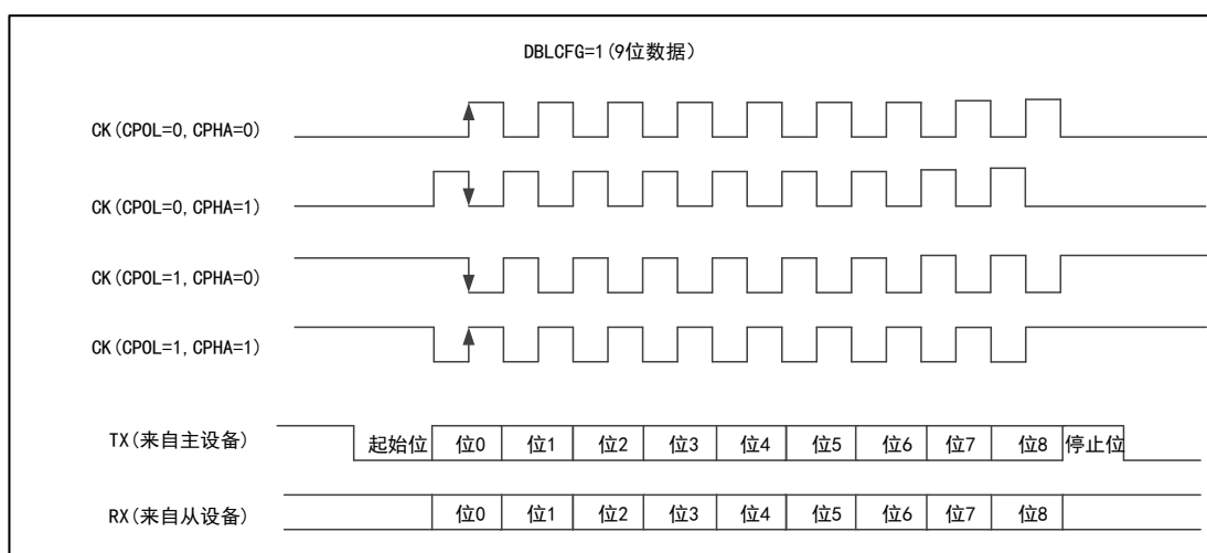
图 96 USART 同步传输时序图 (DBLCFG=1)
