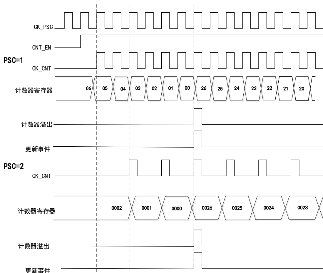
图 27 向下计数模式下，分频因子为 1 或 2 的时序图
