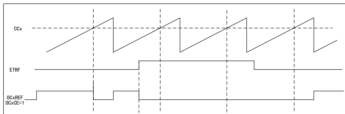
图 87 OCxREF 时序图
