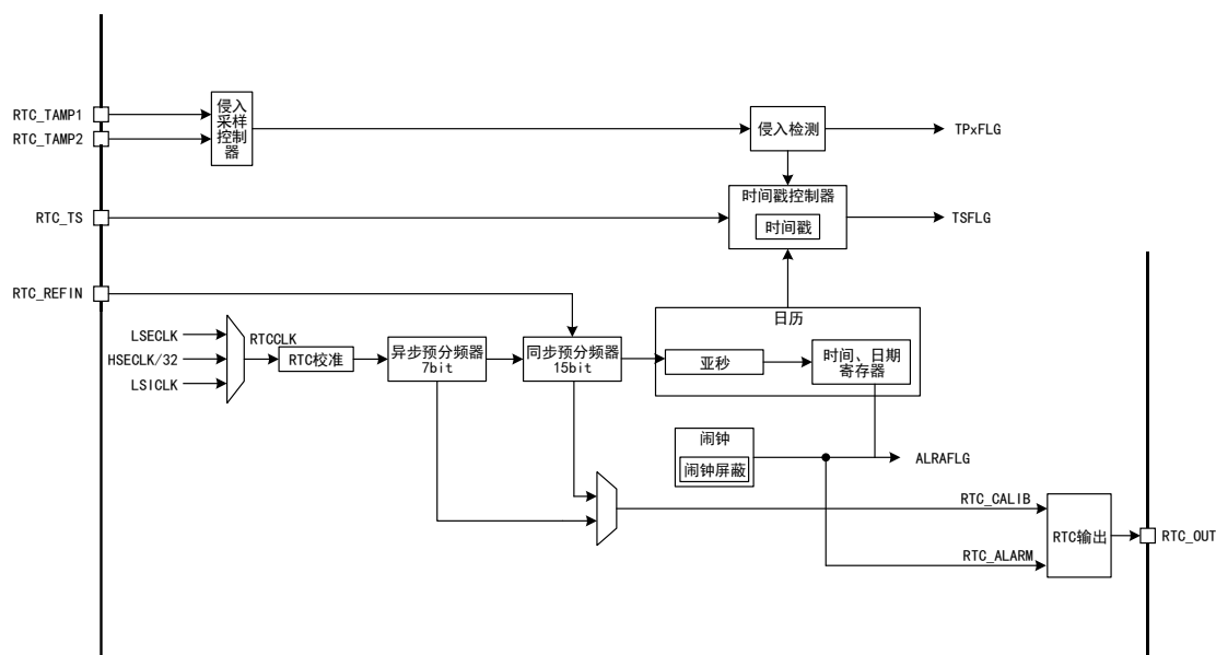
图 91 RTC 结构框图
