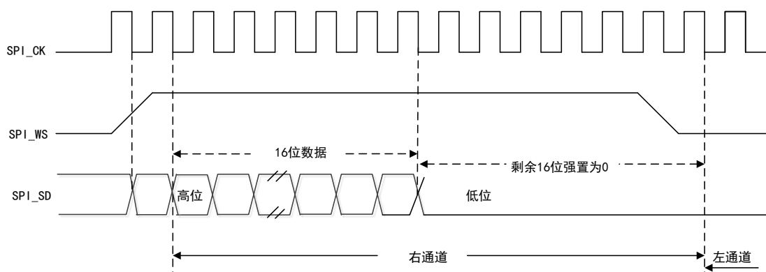
图 115 I2S 飞利浦协议波形（16 位扩展至 32 位）
