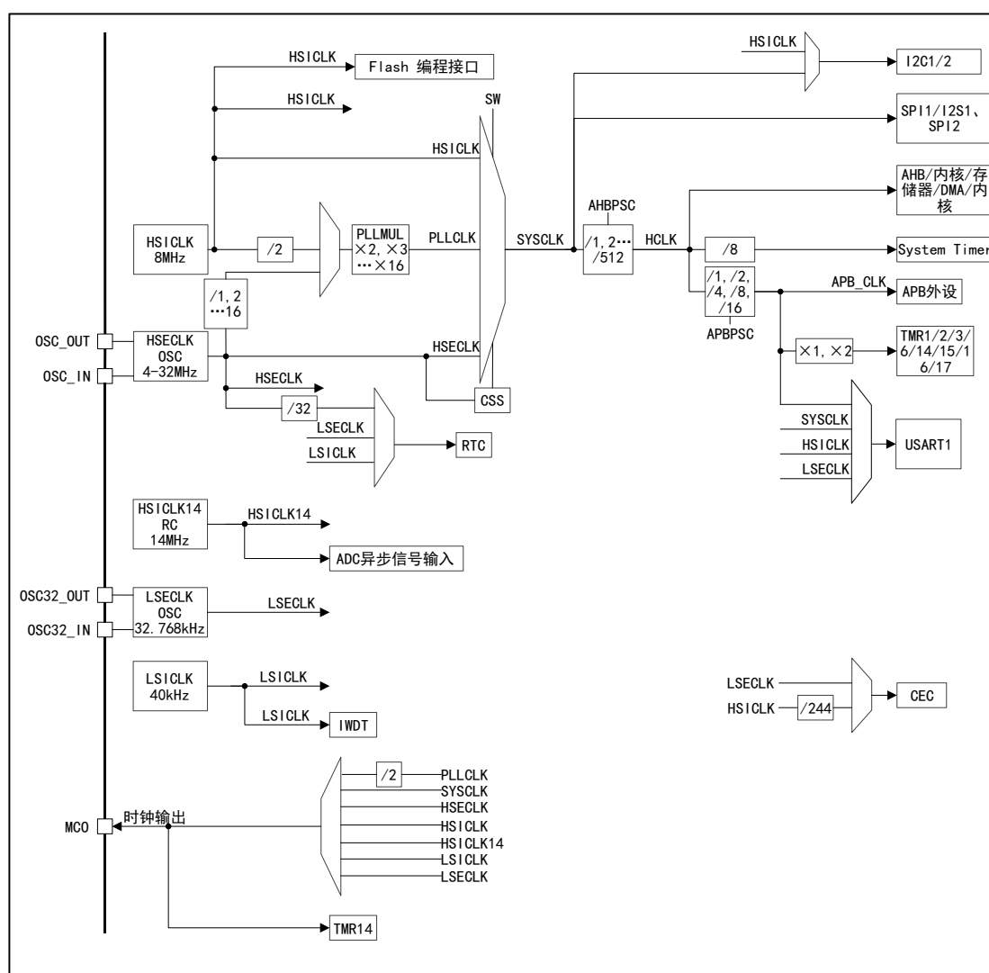
图 4APM32F051x6x8 时钟树
