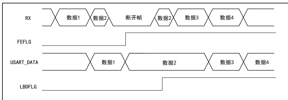
图 98 数据传输状态检测断开帧
